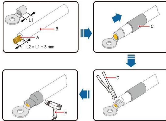
(A) Copper Core Line (B) Insulation layer (C) Heat-shrink tube (D) Hydraulic pliers (E) Hot-air gun
