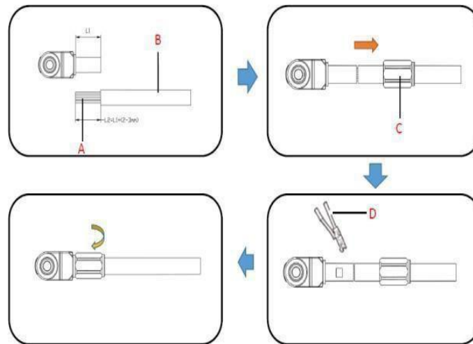
(A) Copper Core Line (B) Insulation layer (C) Protective cover (D) Hydraulic pliers
